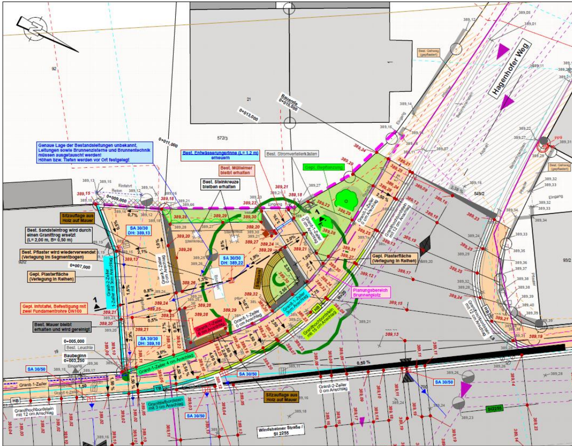
Umgestaltung Bohlenplatz
