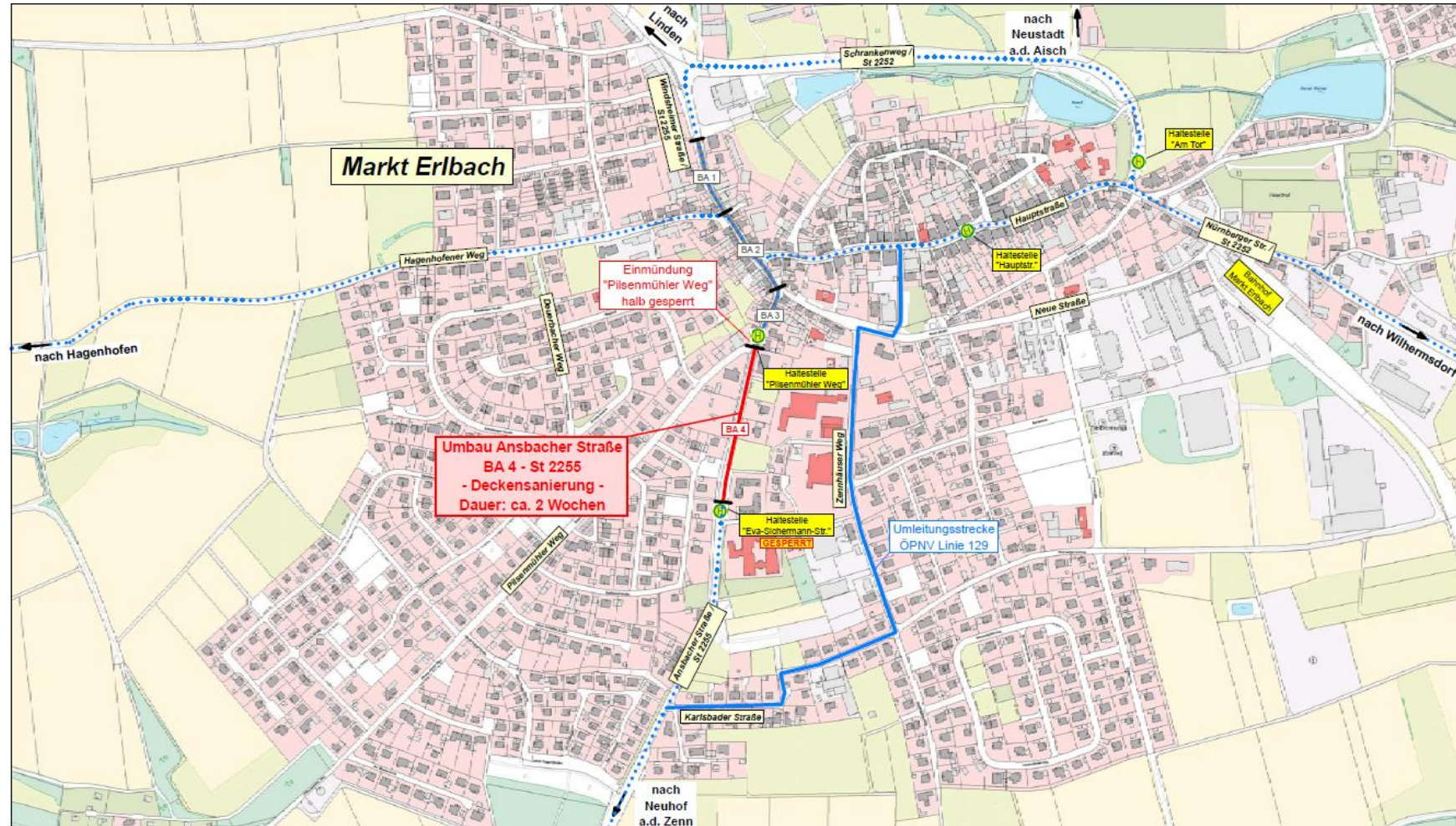
Bauabschnitt 4
